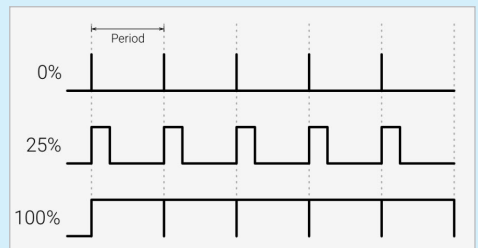
▲ รูปแสดงเปอร์เซ็นต์ของสัญญาณ Pulse
