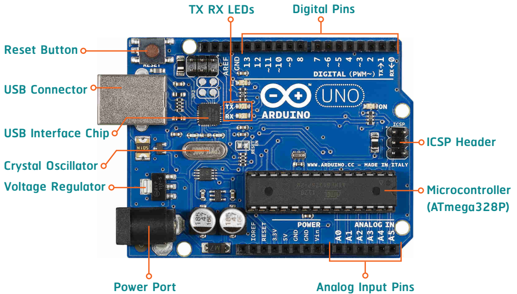
▲ รูปแสดงส่วนประกอบของบอร์ด Arduino UNO Rev 3
